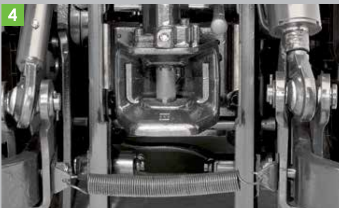
Różne wersje zaczepów, stabilizatorów i łączników centralnych.
